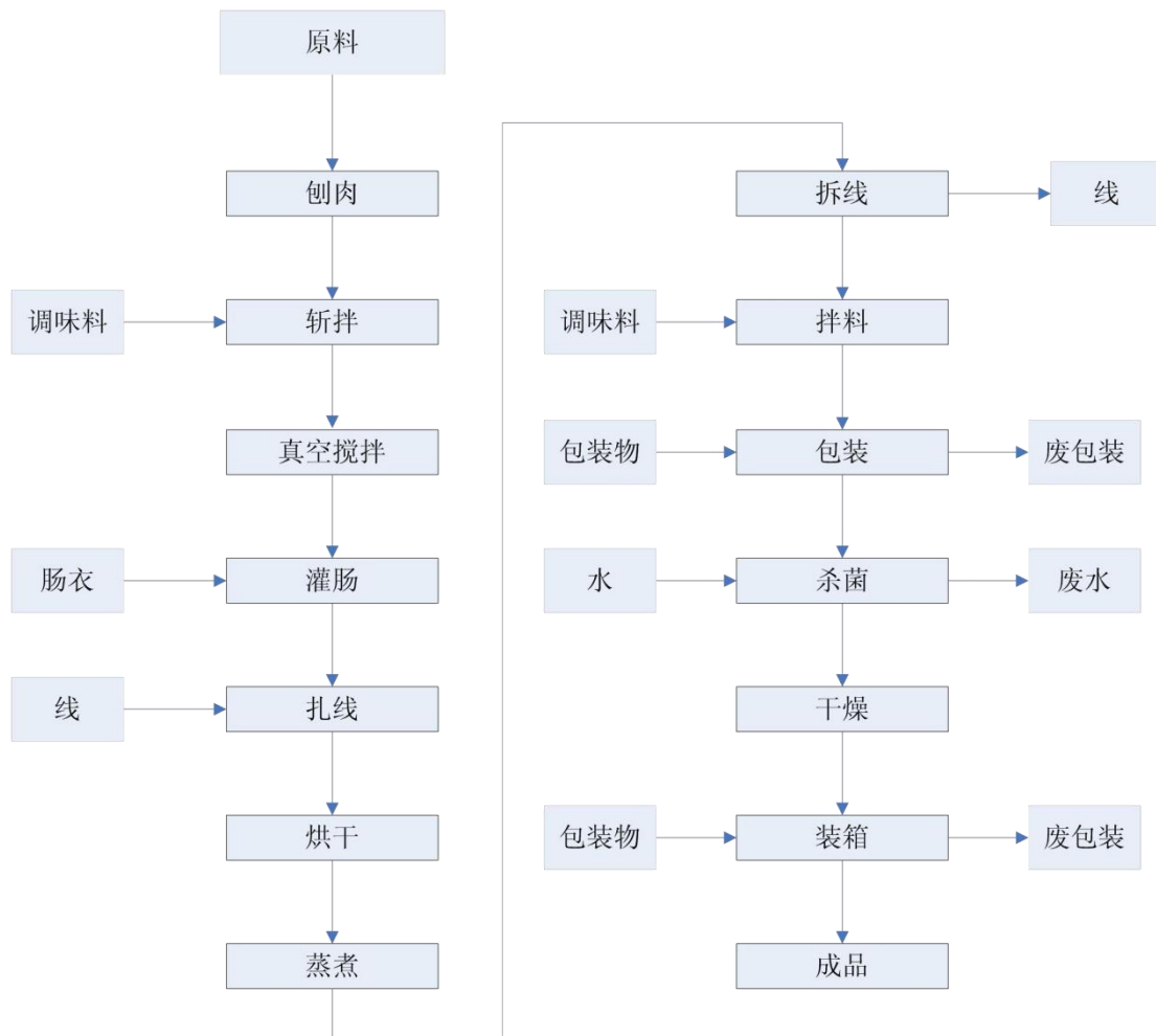
图 6 烤肠生产工艺
