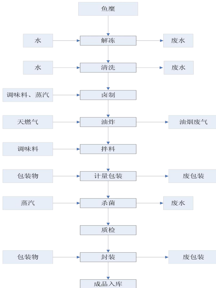
图 4 鱼糜制品生产工艺
